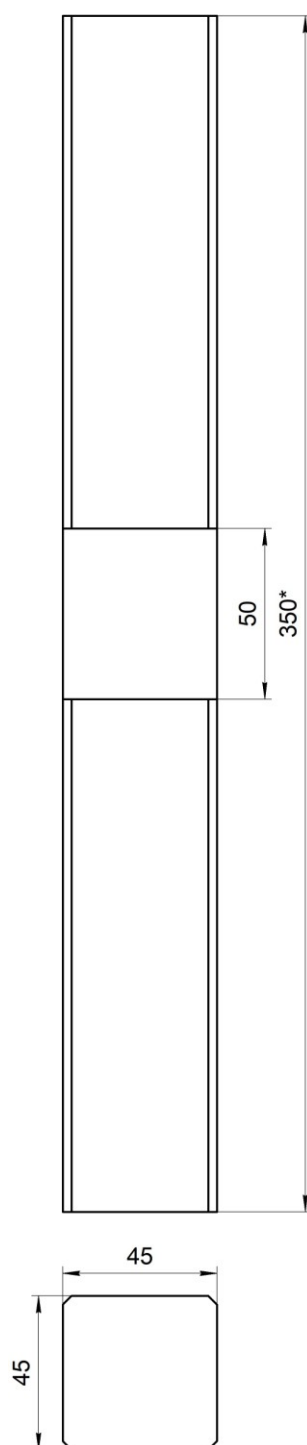
Рис.1 Внешний вид «Указатель лифтовой» НШЕК.468232.206
